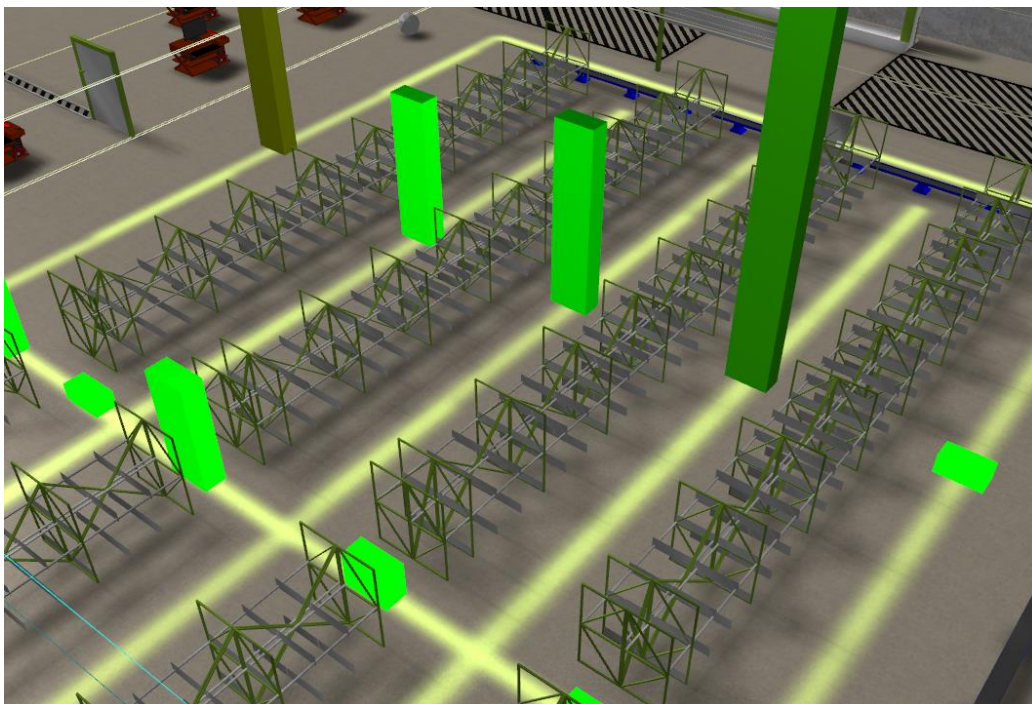
Bild 2: Auslastung von Fahrwegen in 3D-Ansicht
