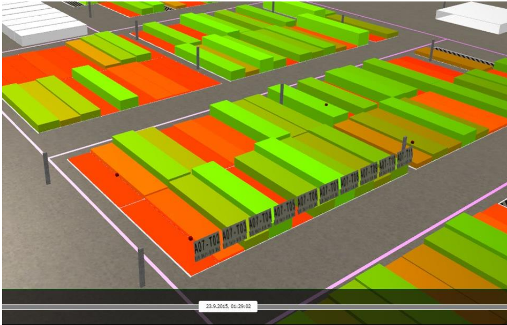
Bild 1: W2MO - Bestandsvisualisierung im Lager in 3D
